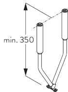
SG 6530 V-Hanger
